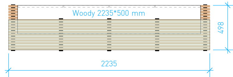
Vue face
