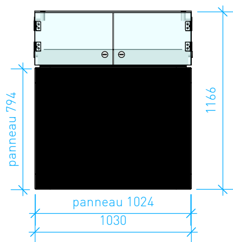
Vue face
