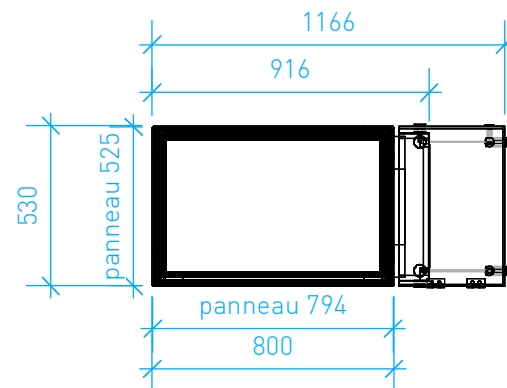
Vue gauche
